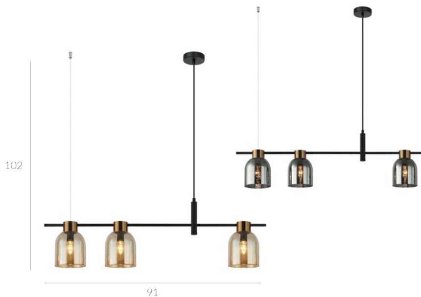
● PND-66892-3-BK-AMB ● PND-66892-3-BK-SG Ø E14 3x40W
